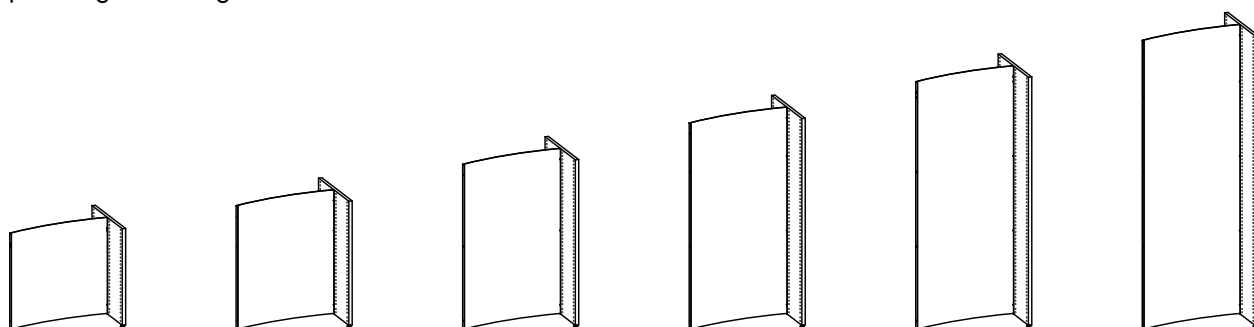
Doppeltseitig Anbauregal - H720/920/1220/1520/1820/2120 mm
