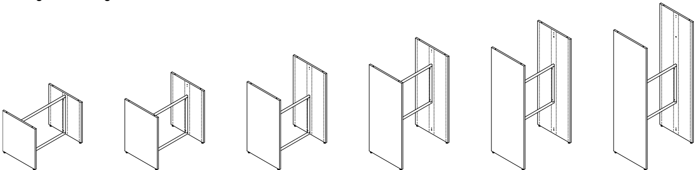
Doppelseitige Grundregal - H720/920/1220/1520/1820/2120 mm
