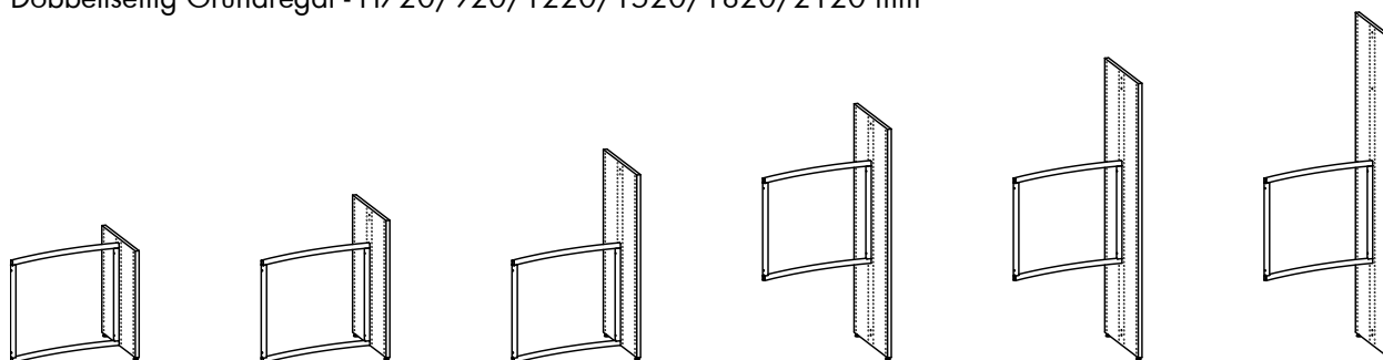
Dobbeltseitig Anbauregal - H720/920/1220/1520/1820/2120 mm
