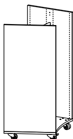
Doppelseitig H1520 mm - 1/2/3 Sektionen
